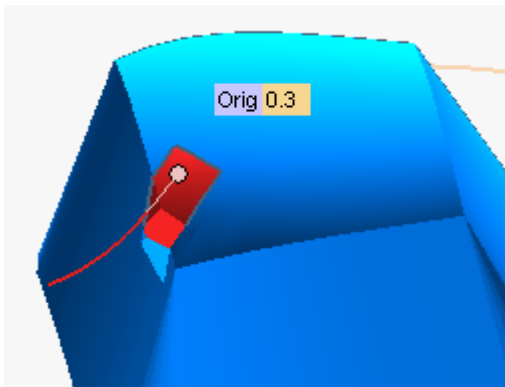
Figura 3. – Modello geometrico/haptic di un pezzo di materiale malleabile sottoposto a lavorazione di asportazione di materiale utilizzando il dispositivo HapticMaster.
